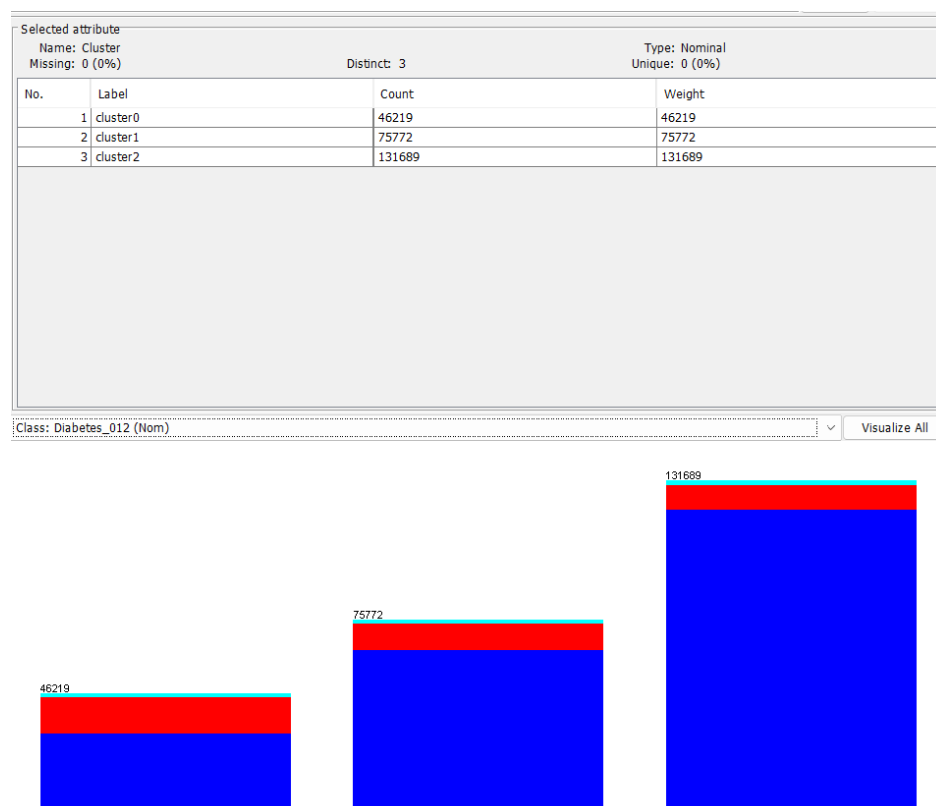
Slika 27 Prikaz klastera u Preprocess panelu
