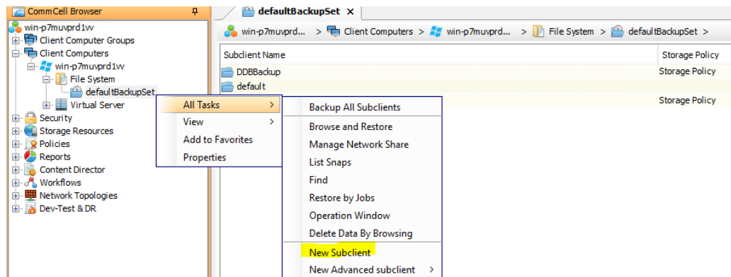
Slika 30. Kreiranje subclienata
