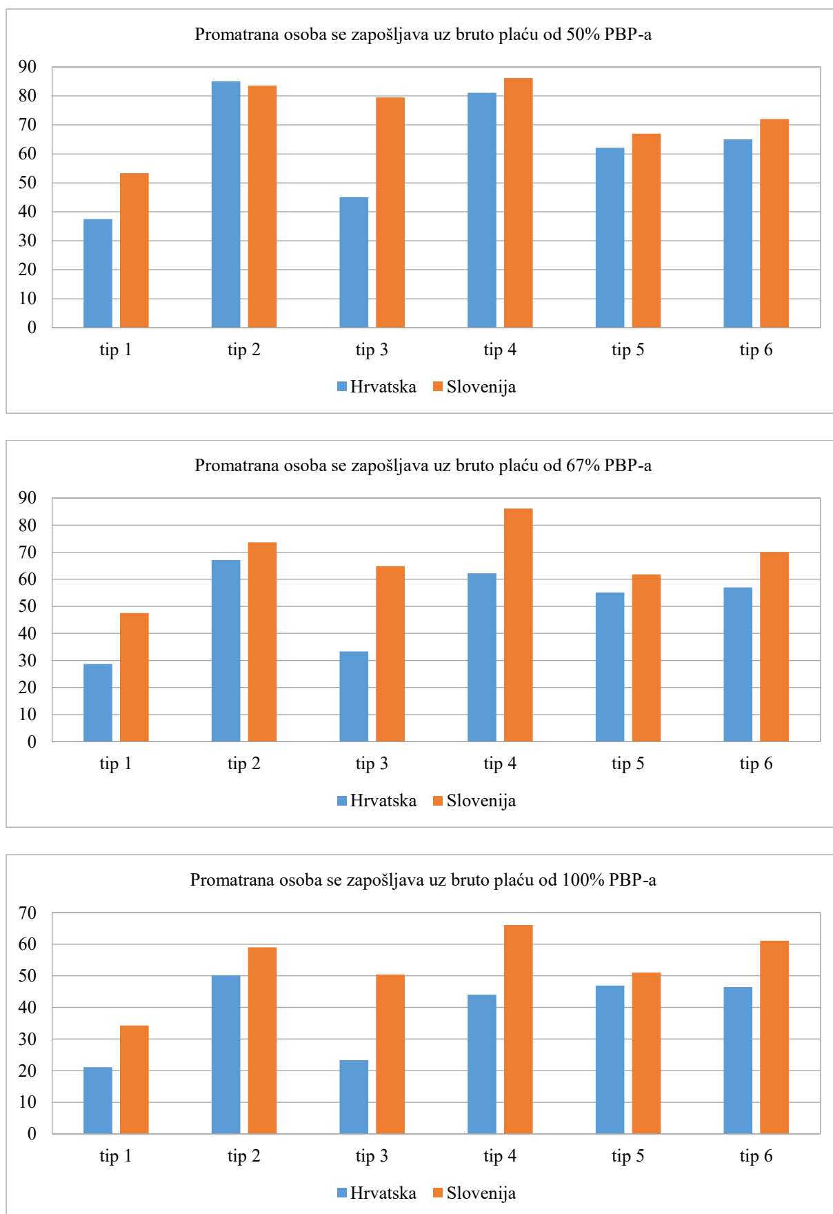
Slika 4.10. Komparativna analiza NSZ-a između Hrvatske i Slovenije u 2017. za odabrane tipove kućanstva na razinama plaća od: (a) 50% PBP-a; (b) 67% PBP-a; (c) 100% PBP-a Izvor: Autorovi izračuni koristeći EUROMOD
