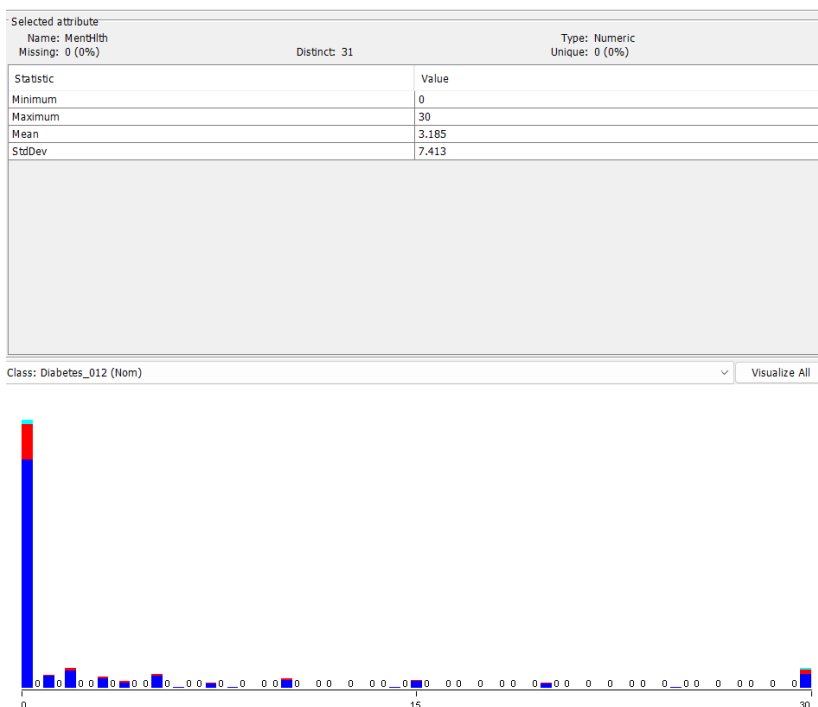
Slika 17 Atribut „MentHlth“
