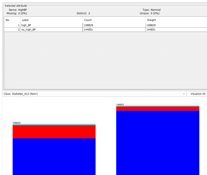
Slika 3 Atribut HighBP
