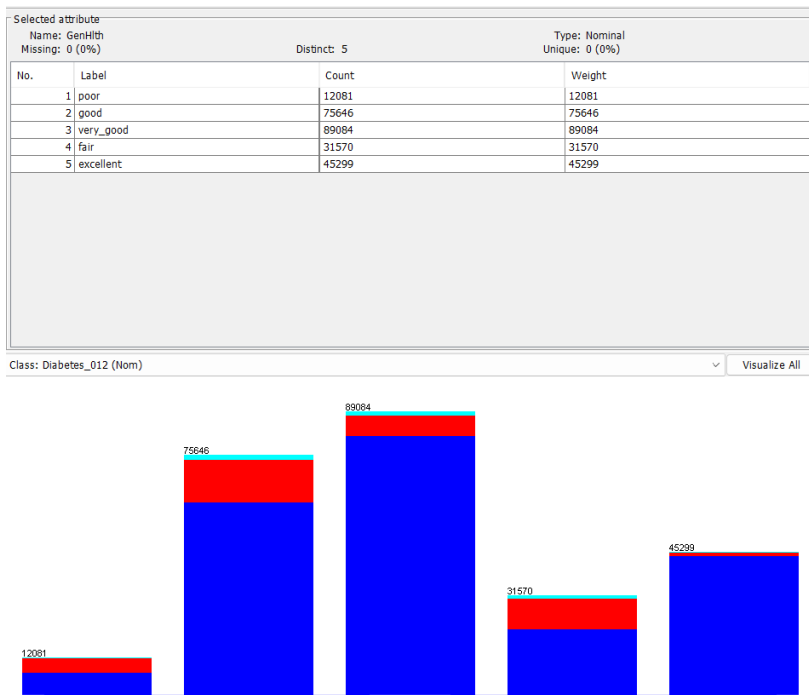
Slika 16 Atribut „GenHlth“
