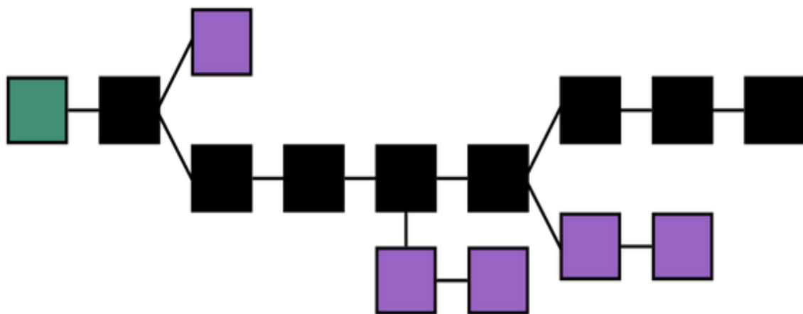
Slika 1. Formacija blockchaina
