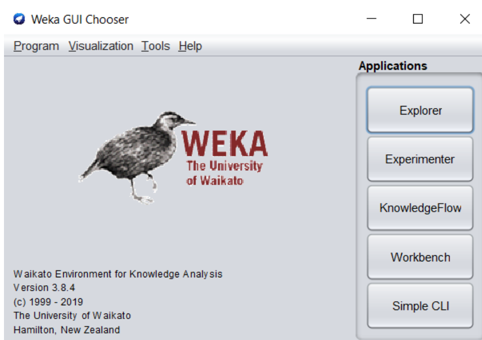
Slika 5 Početni izbornik
