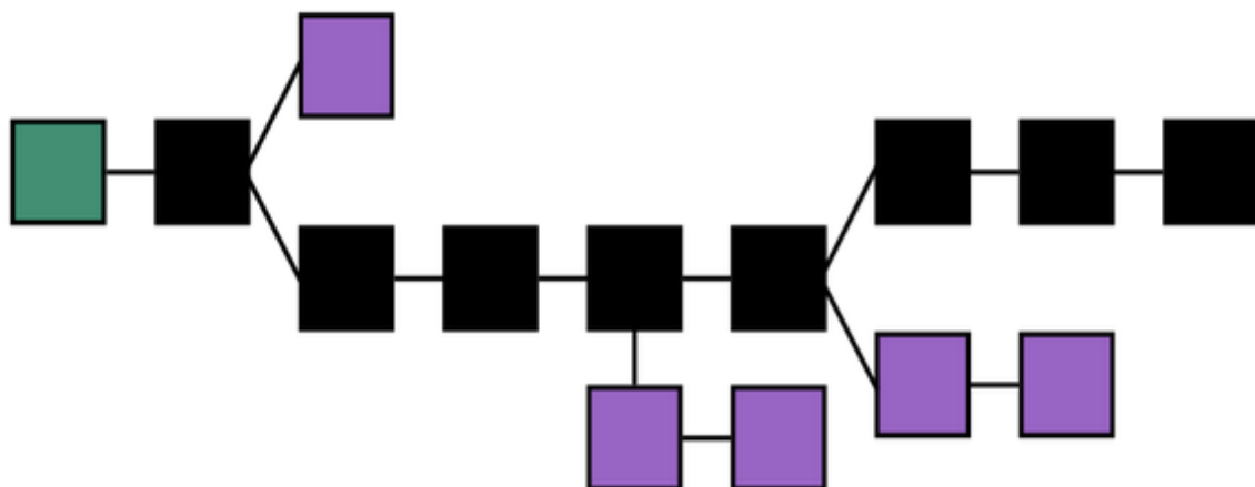
Slika 1. Formacija blockchaina
