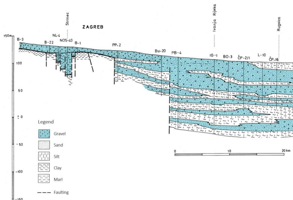
Slika 8. - Shematski hidrogeološki profil zagrebačkog vodonosnika
