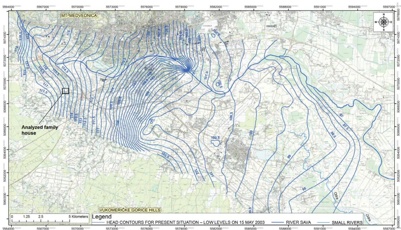
Slika 10. - Konture glave za zagrebački vodonosnik u razdoblju niske razine i lokacija analizirane građevine
