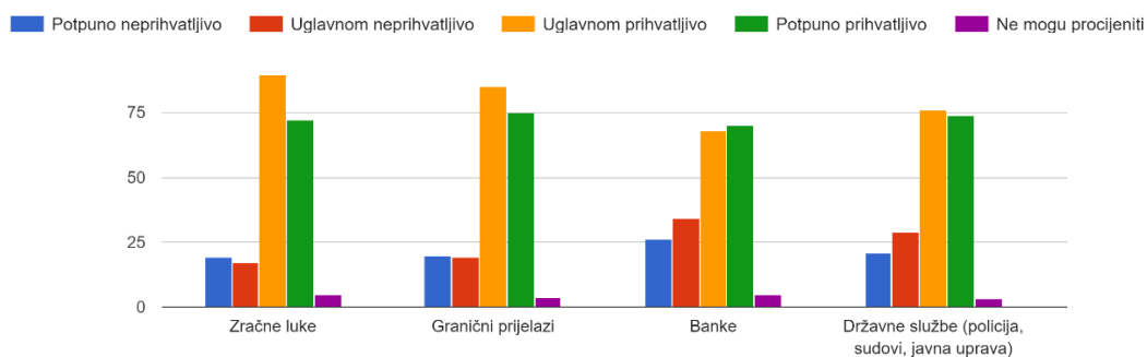
Slika 40: Pitanje 20 (a)
