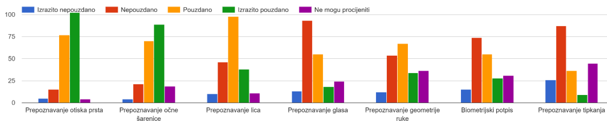
Slika 29: Pitanje 9
