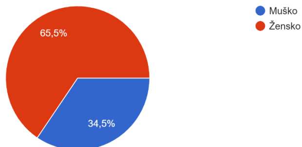
Slika 21: Pitanje 1
